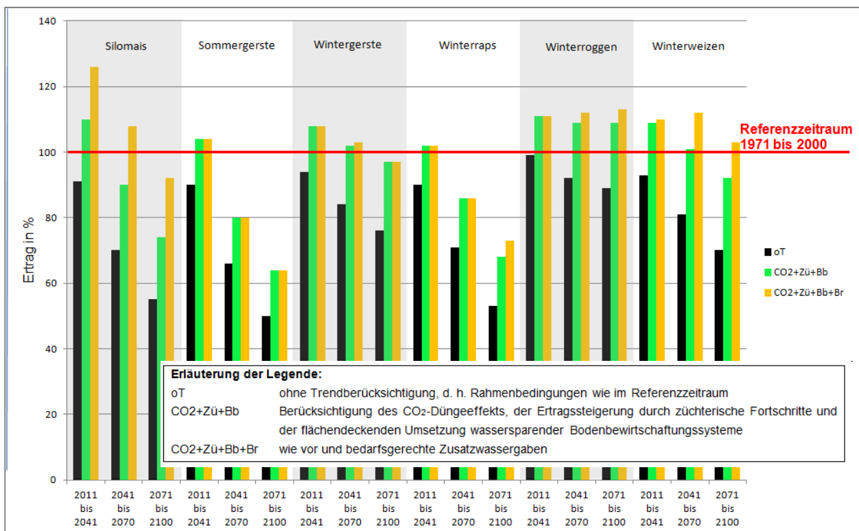
Abb. 2: Übersicht der relativen Ertragsänderungen 2011 bis 2100 für die Landesfläche Sachsen-Anhalts unter Berücksichtigung der unterschiedlichen Trendszenarien in Bezug auf die Ertragssituation im Referenzzeitraum 1971 bis 2000
