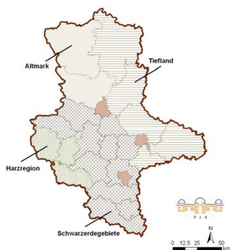
Abb. 10: Gliederung des Landes Sachsen-Anhalt in Boden-Klima-Räume (BKR) (links) sowie (rechts) simulierte Ertragsänderungen (ohne CO 2 -Düngungseffekt, Emissionsszenario A1B, 2071-2100 / 1961-1990) für Winterweizen (WW) und Silomais (SM) in den BKR und Sachsen-Anhalt (leere Zellen: keine valide Modellabschätzung möglich)
