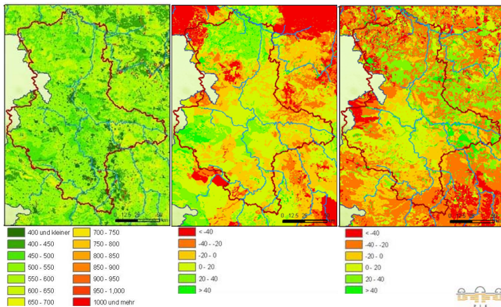
Abb. 6: Simulierte mittlere aktuelle Verdunstung [mm/Jahr] im Zeitraum 1961-1990 (links) und deren Veränderung [%] für den Zeitraum 2071-2100 gegenüber 1961-1990 nach dem Modell WETTREG (Mitte) und REMO (rechts) unter dem Szenario A1B
